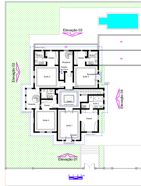
Superior
