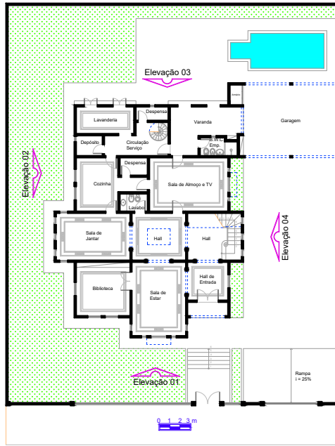
Térreo
