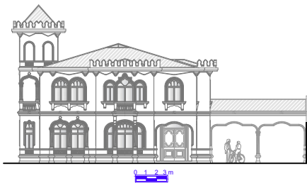
Elevação 01
