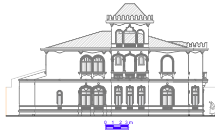
Elevação 02
