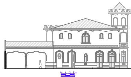
Elevação 03
