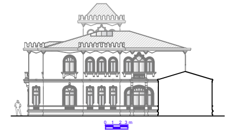
Elevação 04
